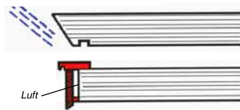
Richtig: Hirnholz geschützt
