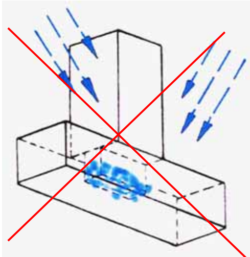
Falsch: unten geschlossen. Wasser kann nicht abfließen, das führt zu Fäulnis am Zapfen.
