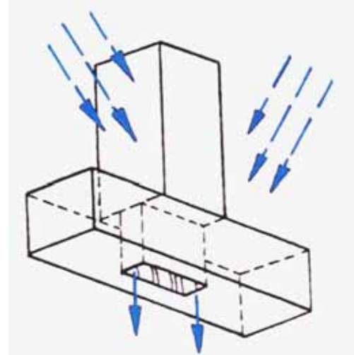
Richtig: unten offen. Wasser kann abfließen.
