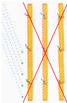
Falsch: Wasser dringt in die Stossfuge ein.
